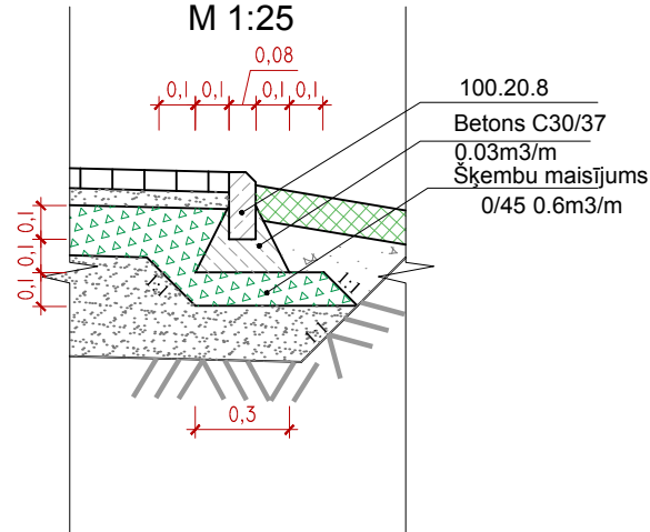
Mezģls 2 M 1:25
