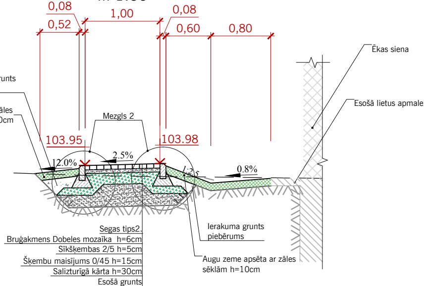
Šķēršprofils 3-3 M 1:50
