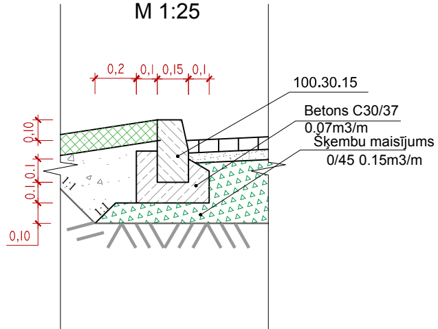
Mezģls 1 M 1:25
