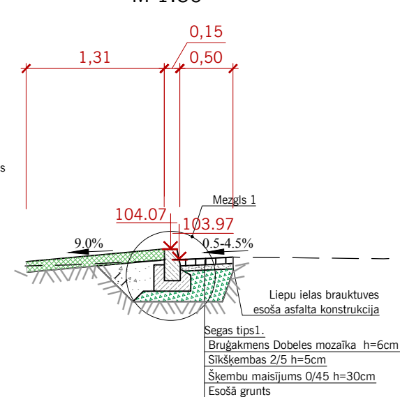
Šķēršprofils 5-5 M 1:50
