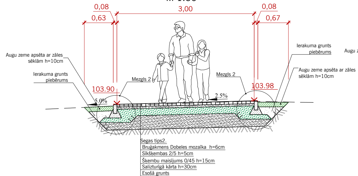
Šķēršprofils 4-4 M 1:50
