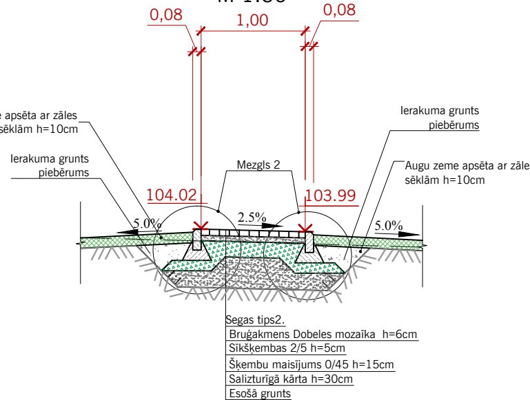
Šķēršprofils 3-3 M 1:50
