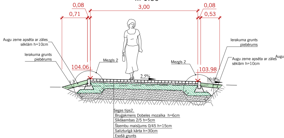
Šķēršprofils 4-4 M 1:50
